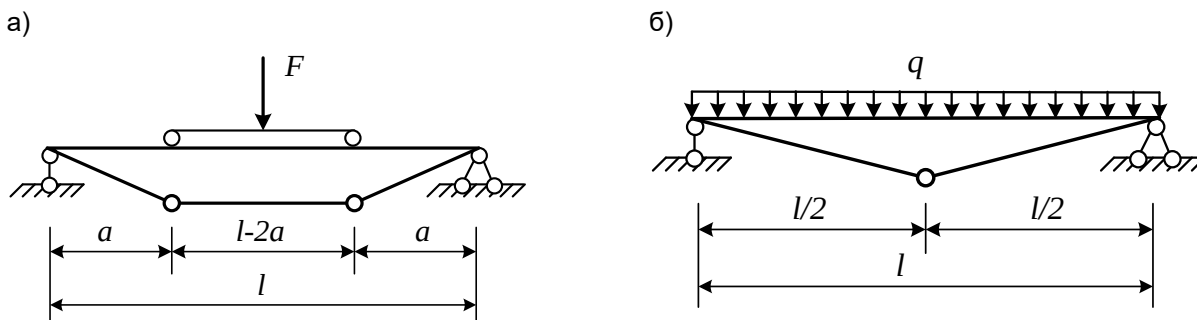
Рисунок 2. Гранична рівновага сталевобетонної балки: а) від дії зосередженої сили; від дії розподіленого навантаження
