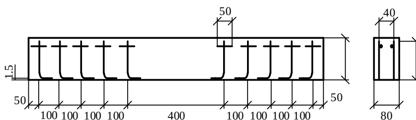
Рисунок 1. Конструкція сталевобетонної балки з анкерами
