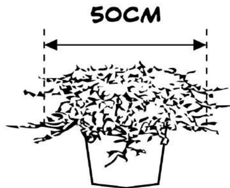
Рис. 5.7. Вимірювання діаметра карликових, ґрунтовкривних, кулястих та середньорослих хвойних рослин
