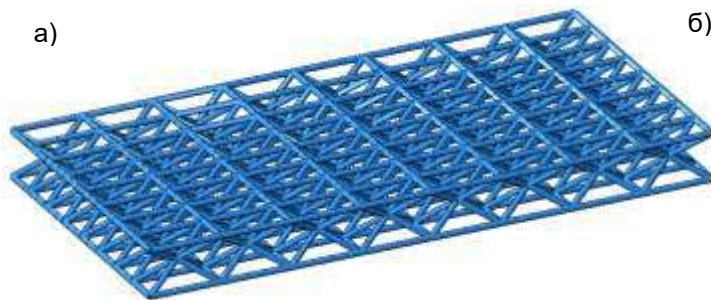
Рис.1 Скінченоелементна схема структурної плити покриття -а; таблиця варіантів висоти структурної плити – б
